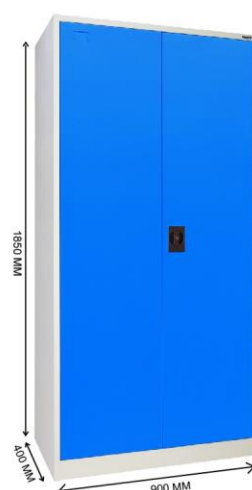
• KF-03S LEMARI BESI DENGAN PINTU BESI AYUN BRUTO 45 KG ■ Blue Package size : H 1880 mm W 940 mm D 75 mm
